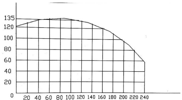
摆臂式90度16寸切割范围图
